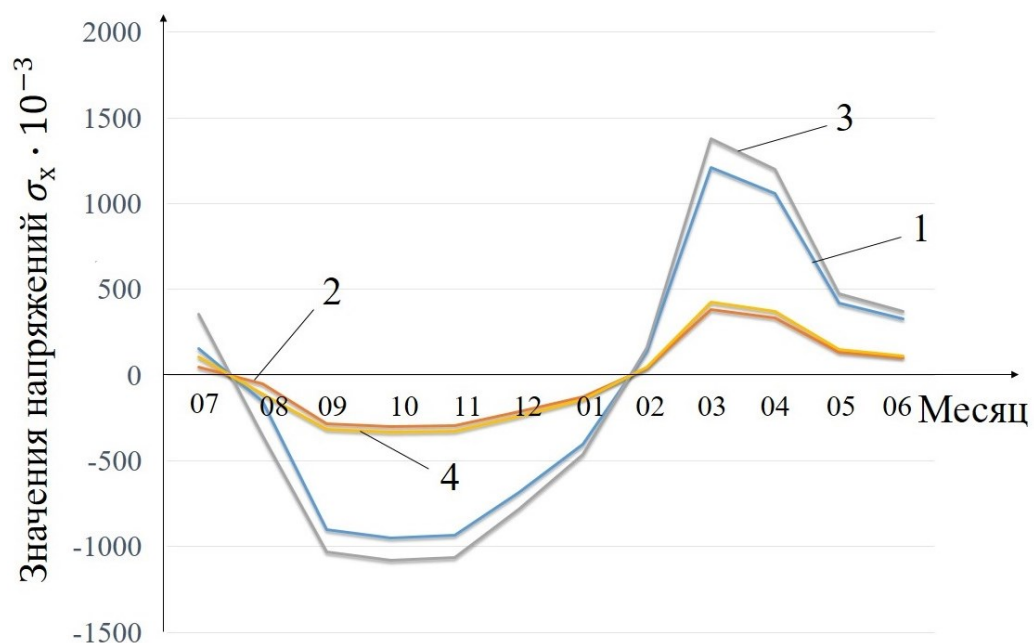
Рис.2. Изменение температурных напряжений в поливинилацетатцементном покрытии в течении года в г. Москве:
